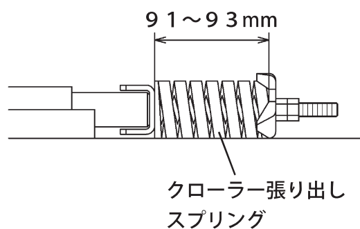
クローラー張り出しスプリング部詳細
