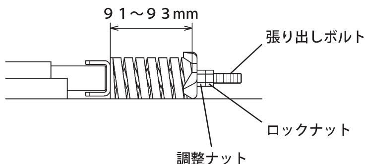
クローラー張り出しスプリング部詳細
