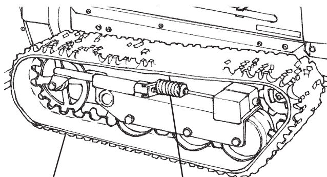
クローラー クローラー張り出しスプリング
